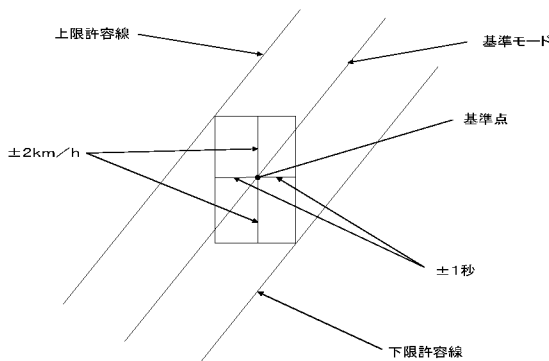
図 1: 10モード燃費の速度パターン
